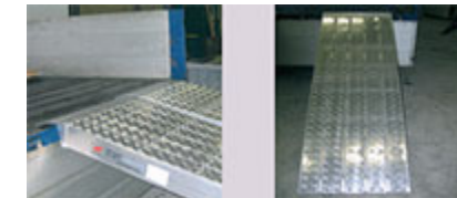
Schwerlaststrampen ohne Rand, Traglast 4000 bis 17500 kg / per Paar
